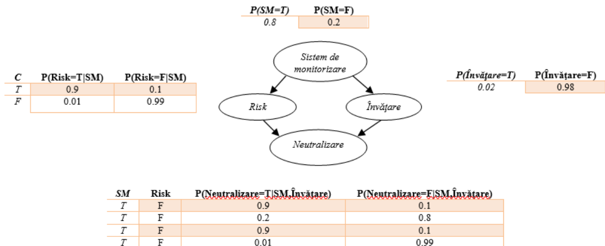
Figura 1. Reprezentarea rețelei bayesiene
